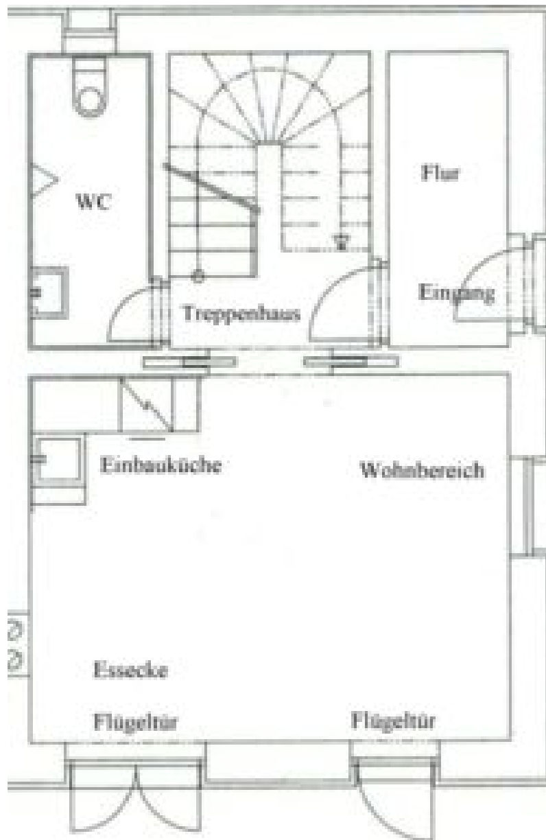
Grundriss der rechten Wohneinheit Paterre/Erdgeschoss.
